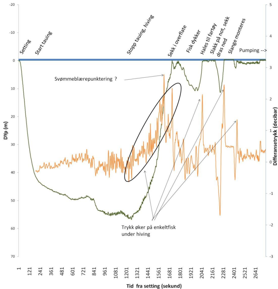
Figur 2.1.1. Trykkforløp i sekk på individuell fisk i et 11 tonn snurrevadhål med pumping som ombordtakingsmetode (fra "Bernt Oskar"). Grønn kurve er dybde på sekk, mens oransje kurve er forskjell mellom omgivelsestrykk (differansetrykk) og trykk inne i en vannfylt blåse montert inne i sekk (Ingolfsson m.fl. 2001). Fra start av tauing med økende fangst til stopp tauing er det en gradvis økning i trykk utover omgivelsestrykk. Ved hiving øker trykk på enkeltfisk. Dette skjer gjentatte ganger når fisk blir tatt til overflate etter dykking (ved dykking reduseres trykk utover omgivelsestrykk). Et fall i differansetrykk før sekk er i overflate kan være effekt av svømmeblærepunktering. Metode for trykkmåling på fisk bør undersøkes nærmere i fremtidige forsk.
